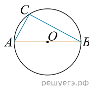
Градусна міра вписаного кута ACB
