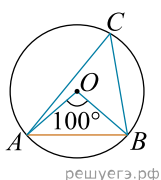
Градусна міра вписаного кута ACB
